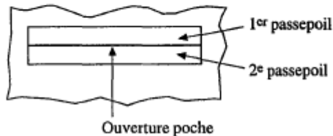
3 - Poche à deux passepoils
