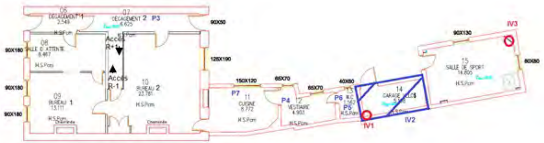
Ancien Bureau de Police - ESCAUDAIN (RdC)
